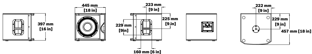
Abbildung 7.4: ELX200-12S-Abmessungen
