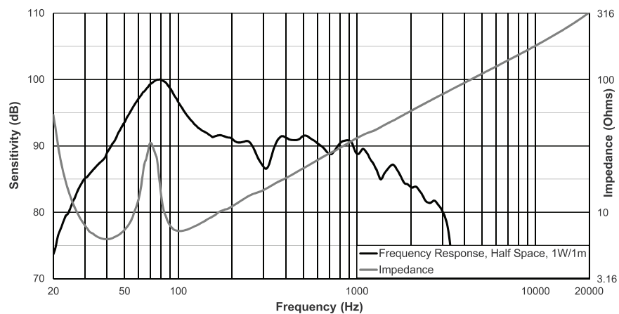
Abbildung 7.10: ELX200-18S Frequenzgang und Impedanz
