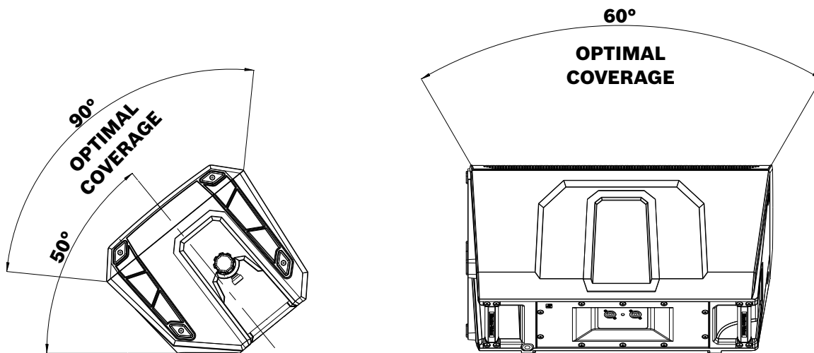
Abbildung 3.2: Optimaler Abstrahlwinkel in Monitorposition (seitliche Ansicht von links und Vorderansicht von rechts)
