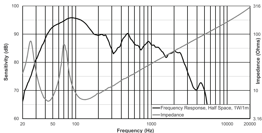
Abbildung 7.9: ELX200-12S Frequenzgang und Impedanz
