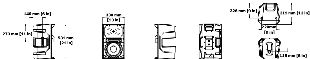
Abbildung 7.1: ELX200-10-Abmessungen
