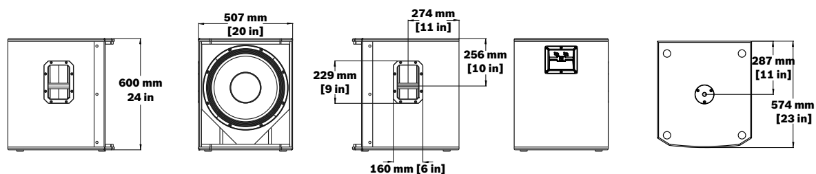
Abbildung 7.5: ELX200-18S-Abmessungen
