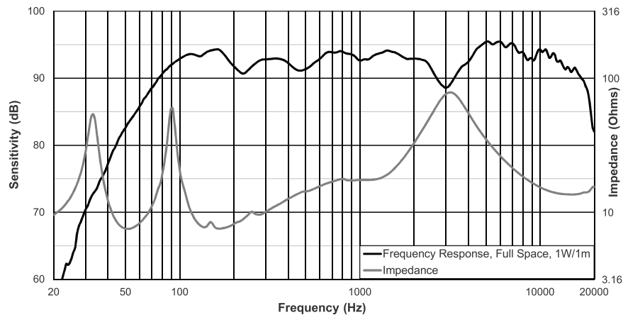
Abbildung 7.7: ELX200-12 Frequenzgang und Impedanz
