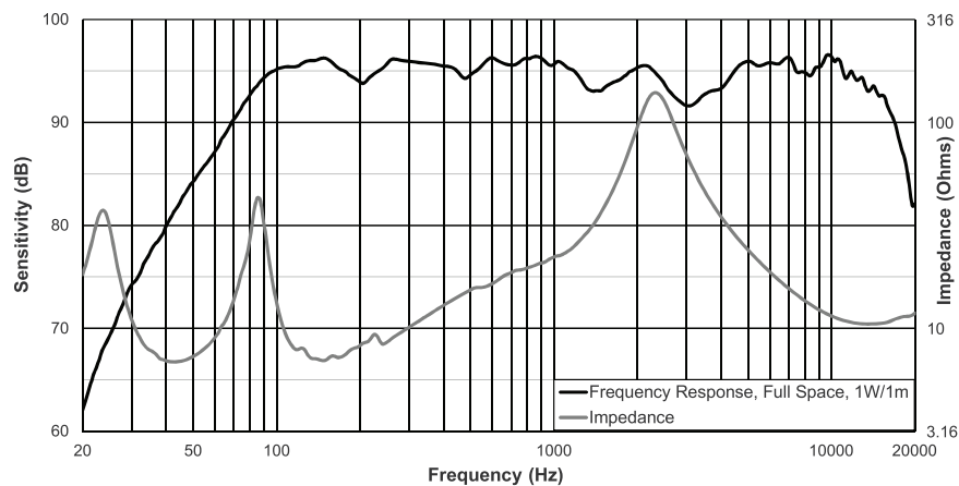
Abbildung 7.8: ELX200-15 Frequenzgang und Impedanz
