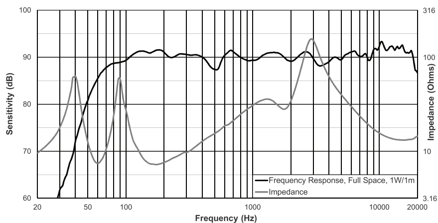
Abbildung 7.6: ELX200-10 Frequenzgang und Impedanz
