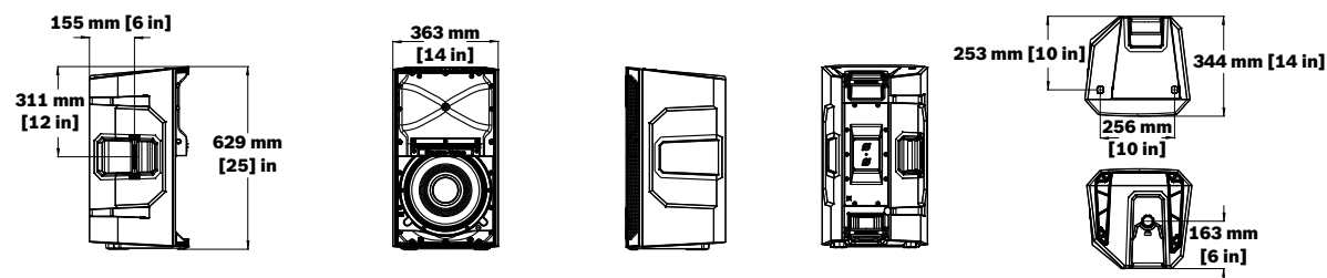
Abbildung 7.2: ELX200-12-Abmessungen
