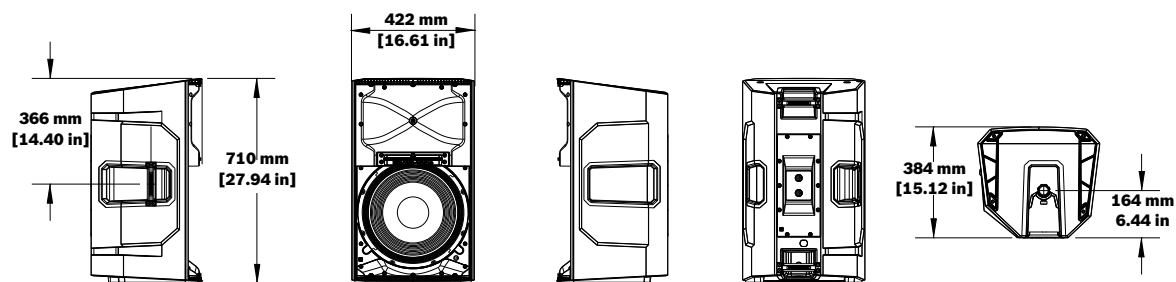
Abbildung 7.3: ELX200-15-Abmessungen
