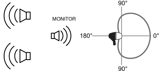
Ubicaciones recomendadas para altavoces con micrófonos de cardioide
