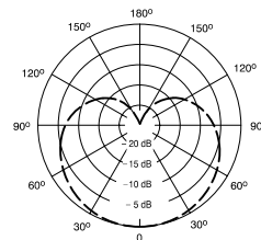
Courbe de directivité typique
