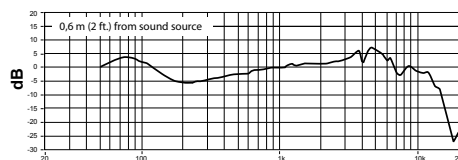
Réponse en fréquence typique
