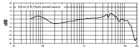
Typischer Frequenzgang
