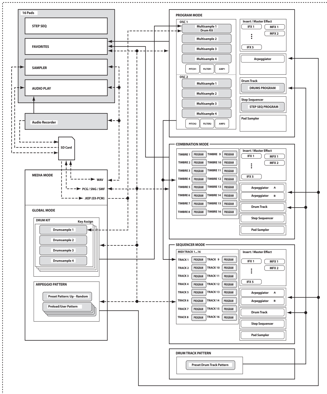
Beziehungsdiagramm der KROSS-Modi
