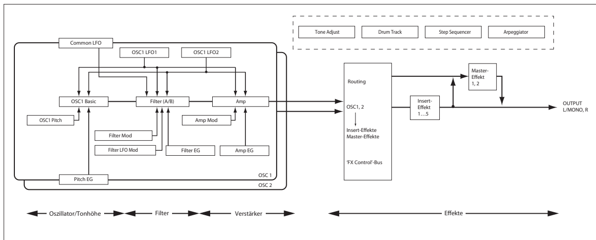
Aufbau eines Programs
