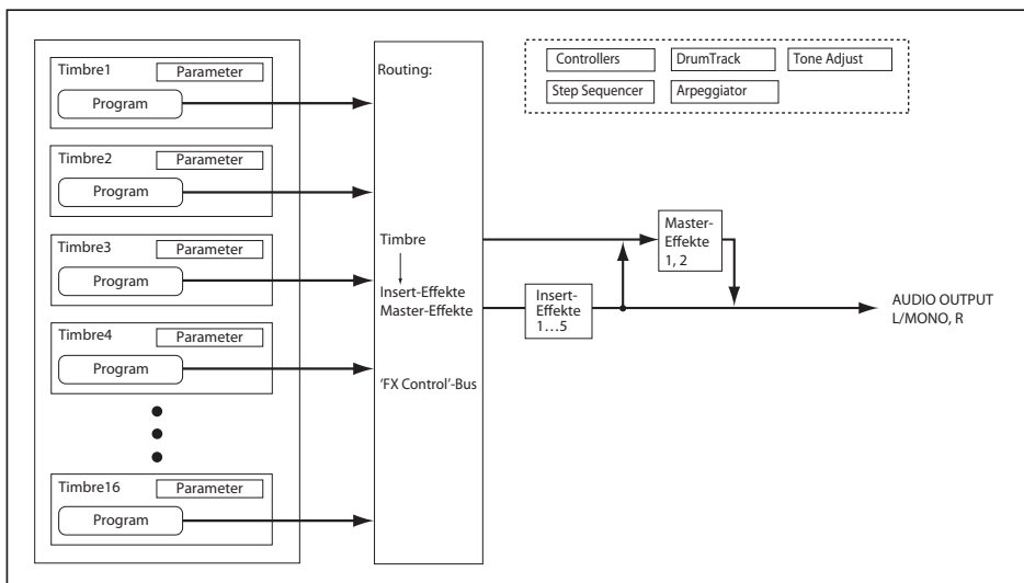
Aufbau einer Combination und zugeordnete Display-Seiten
