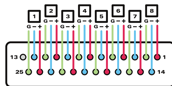
Pinbelegung Sub-D 25-poliger Anschluss
