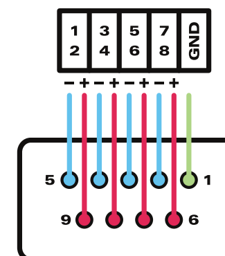
Pinbelegung Sub-D 9-poliger Anschluss
